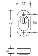
Schutzrosette mit Zylinderabdeckung 316...Z...
