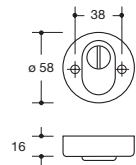
Schutzrosette mit Zylinderabdeckung 306...Z...
